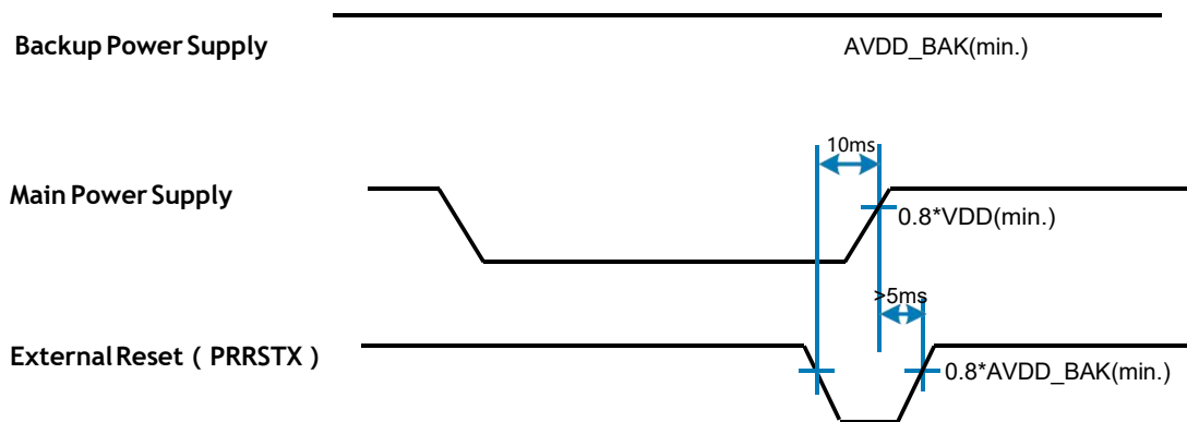
图 4 上电时序
