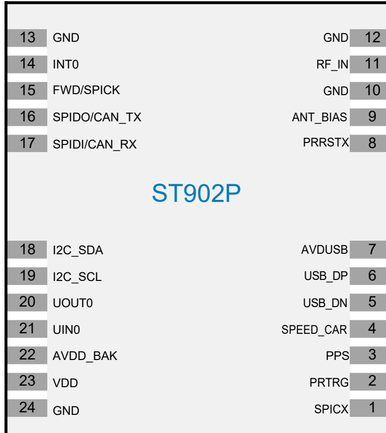
图 2 引脚分布图
